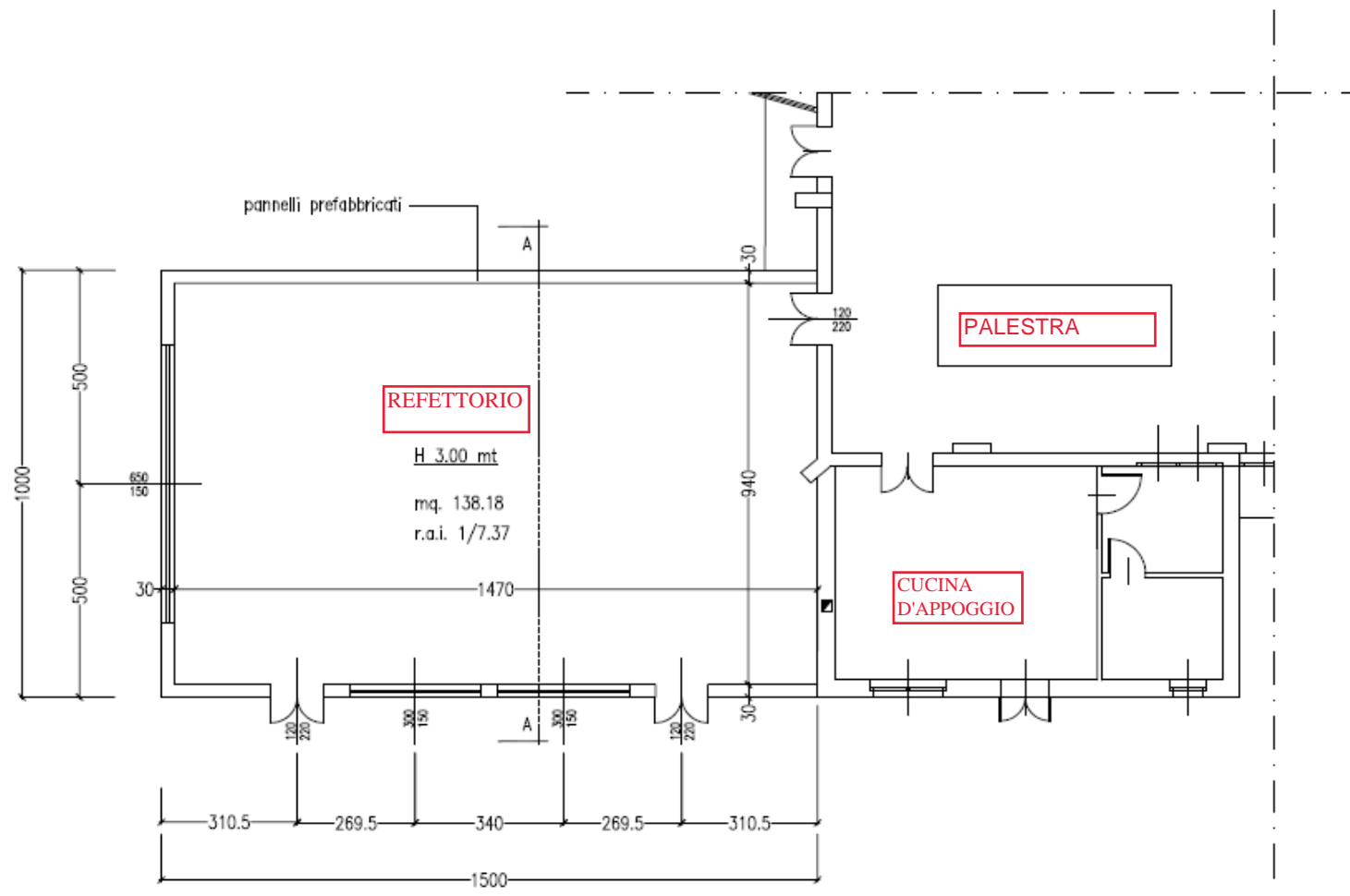
PIANTA PIANO TERRA scala 1:100
